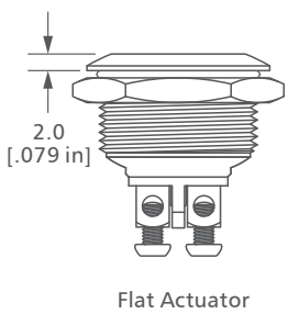
Flat Actuator
