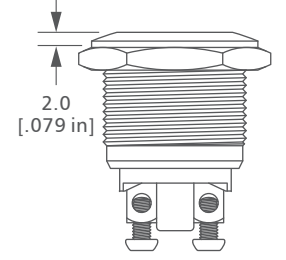
Flat Actuator
