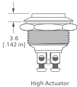
High Actuator
