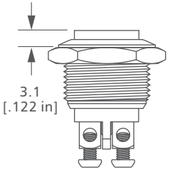
High Actuator
