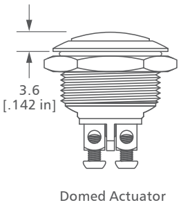
Domed Actuator
