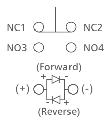
SPST Illum.
