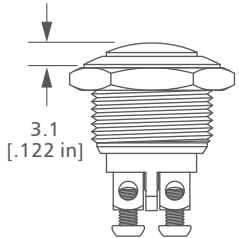
Domed Actuator
