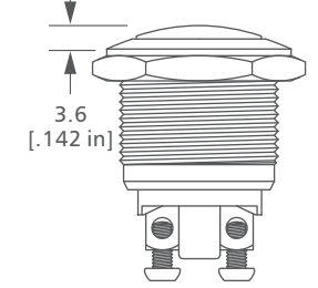
Domed Actuator
